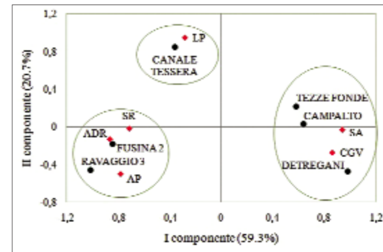
Fig. 2. Ordinamento simultaneo delle sei barene e dei sei habitat, ottenuto dall'applicazione dell'analisi delle componenti principali (PCA) alla matrice dei valori di superficie (ha). (●) Barena; (♦) Habitat. Il primo asse spiega il 59,3% della variabilità totale, mentre il secondo asse il 20,7%. Legenda: ADR = argine/dosso con vegetazione ruderale; SA = aree con vegetazione alofila a dominanza di Salicornia , LP = aree con vegetazione alofila a dominanza di Limonium/Puccinellia/Aster/Juncus/Spartina , SR = aree con vegetazione alofila a dominanza di Sarcocornia/Halimione , CGV = chiari, ghebi, velme interne, AP = aree pianeggianti poco o per niente vegetate.
